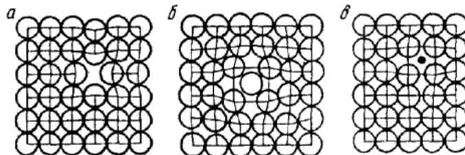
Рисунок 1.3 – Точечные дефекты в кристаллической решетке:
